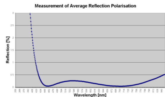
Figura 13 - La reflectividad del revestimiento antirreflectante depende de la longitud de onda de la señal (EDM).
