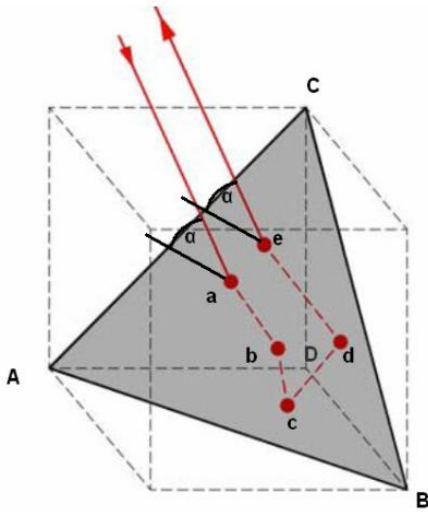
Figura 10 - Ruta de los rayos entrante y saliente en un prisma triple.
