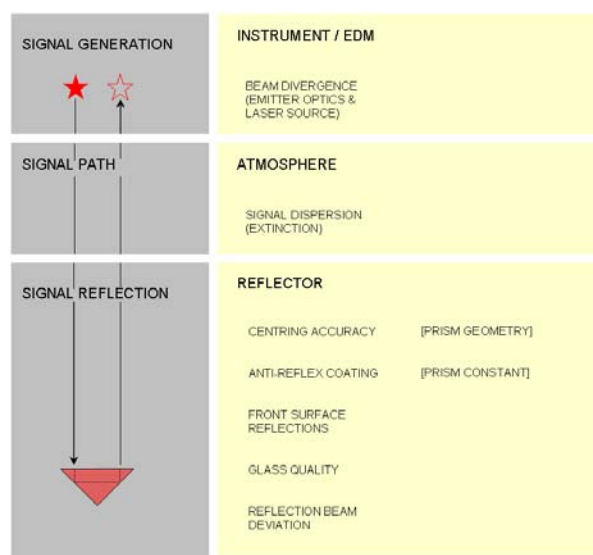
Figura 1 – Diferentes fases de una medición electrónica de distancia.
